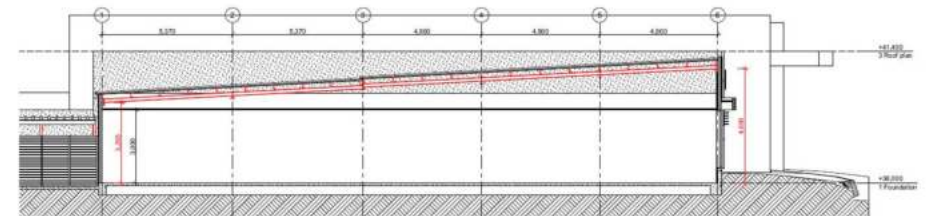
01 Section A-A Scale 1:100
